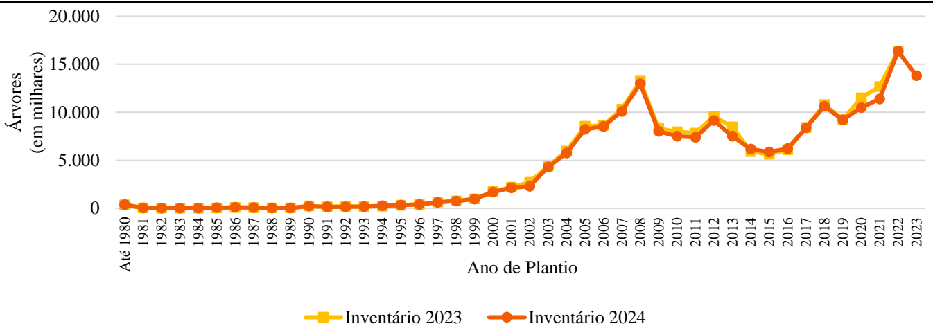
Gráfico 9 – Laranjas: Árvores por ano de plantio do talhão, replantas não incluídas [inventários de 2023 e 2024]
