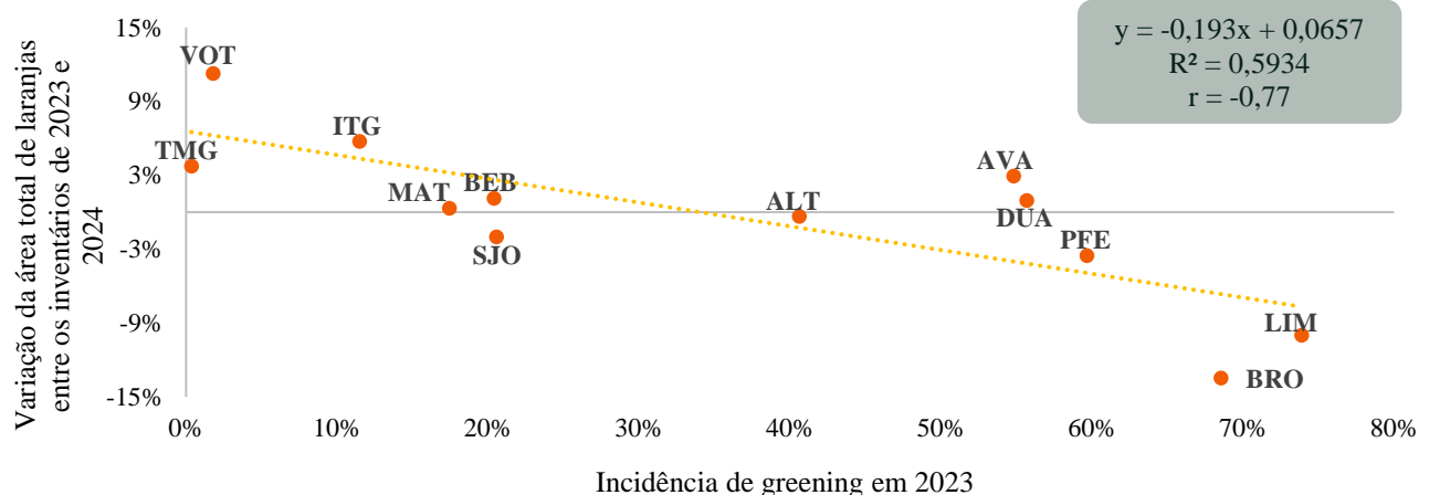
Gráfico 5 – Laranjas: Correlação negativa entre a incidência de greening e a variação da área de laranjas em cada região entre os inventários de 2023 e 2024 [inventário de 2024]
