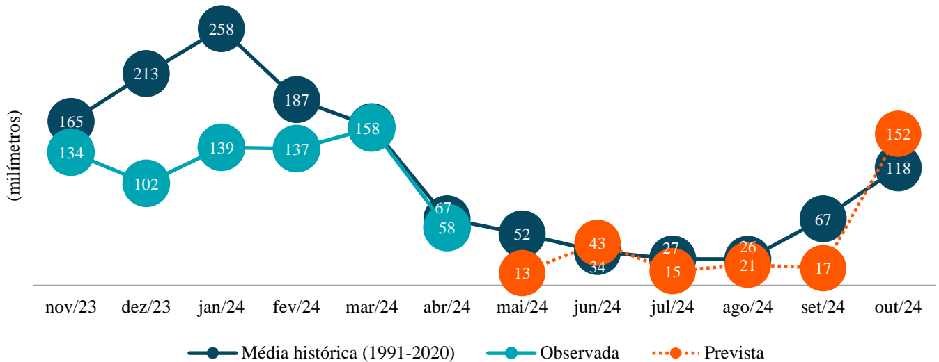
Gráfico 5 – Precipitação observada de novembro de 2023 a abril de 2024 e previsão de maio a outubro de 2024
