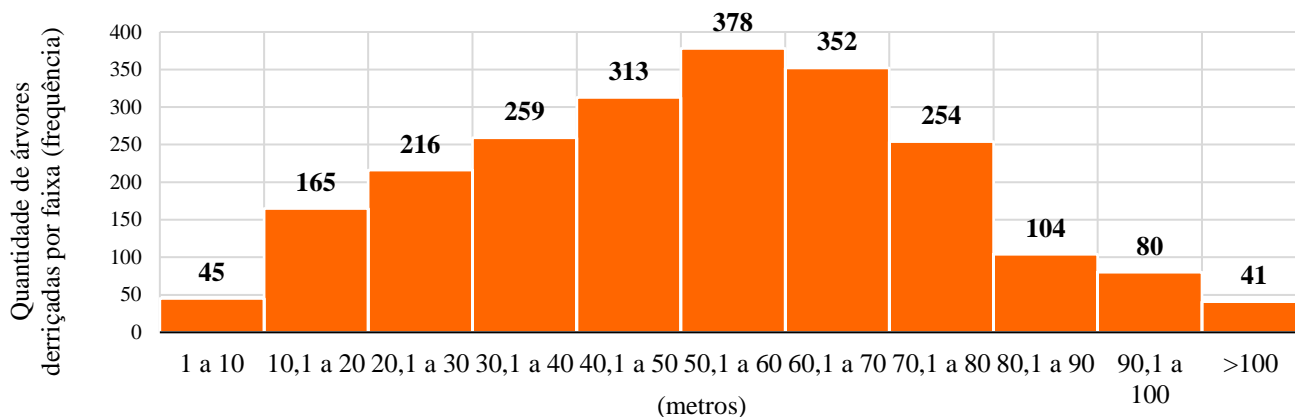
Gráfico 9 – Histograma das distâncias entre a árvore derrçada e a borda mais próxima do talhão
